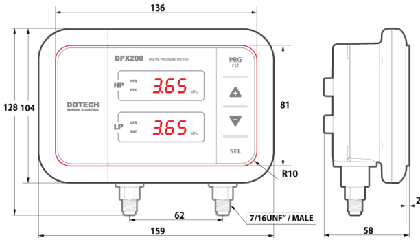
LP : 저압센서 | HP : 고압센서 (단위 : mm)
